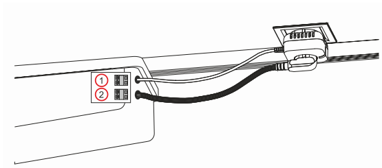
1 - Klemmen des Eingangs für die Bedienung des Umrichters (potentialfreier Kontakt); 2 - Klemmen für die Stromversorgung des Umrichters mit 230 V
